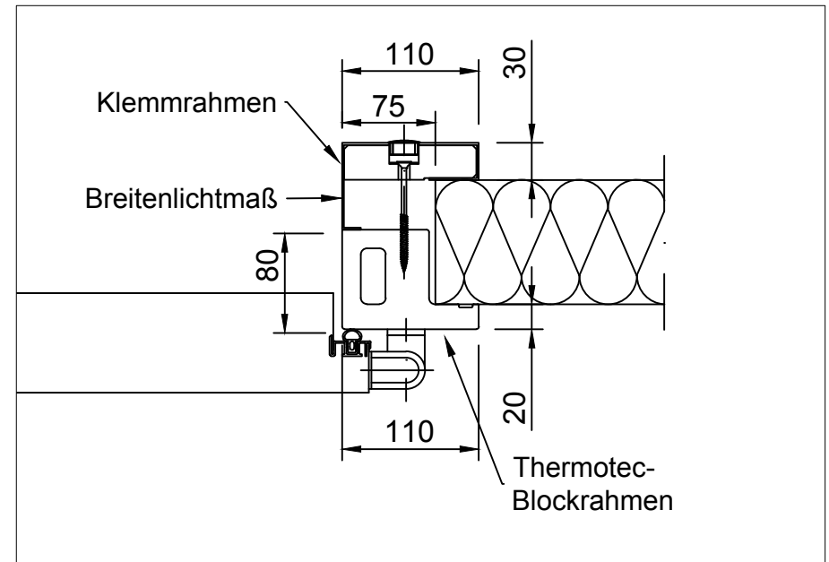
Detail X Maßstab 1:5
