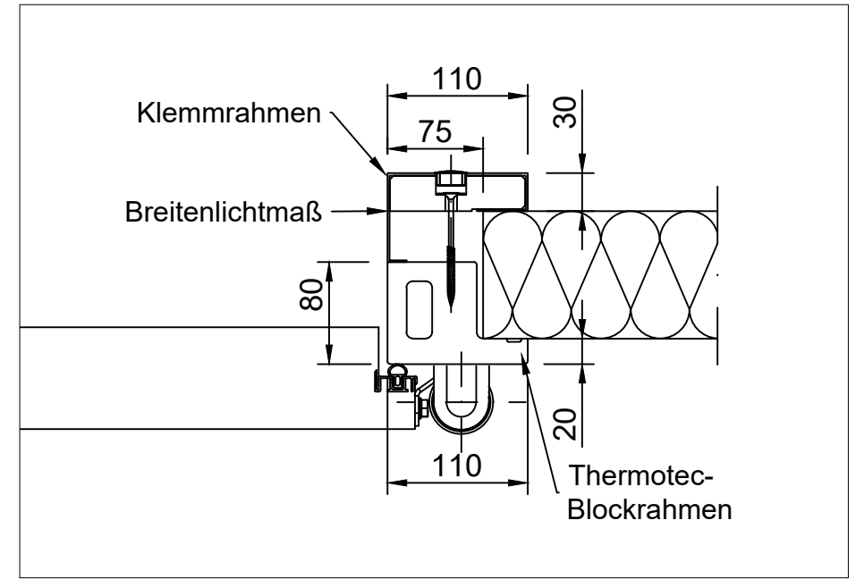
Detail X Maßstab 1:5
